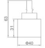
Cartucho termostático con regulador de temperatura 40 Cartridge 40mm with temperature ring
